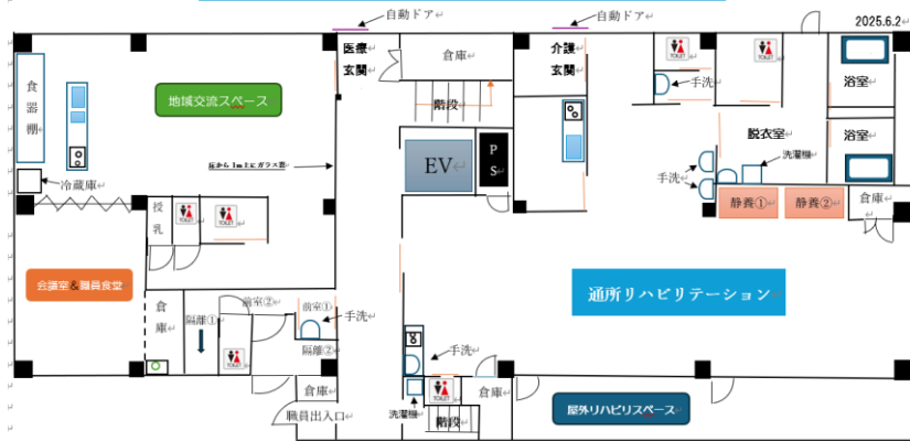
新相川診療所・併設事業所建設（平面図）1 階
